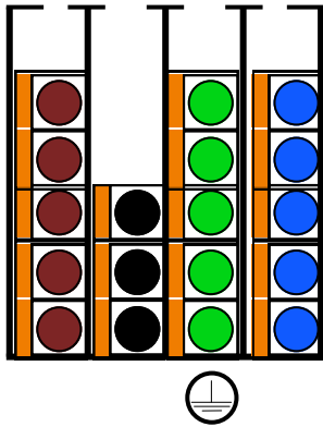
Light & Loop + Timer Overrun Extractor Fan
